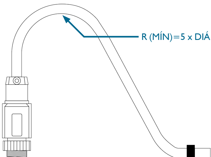
INSTALACION FIJA
